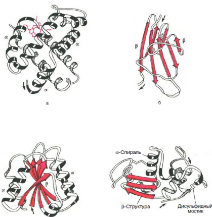
Рис.2. Доменное строение глобулярных белков
