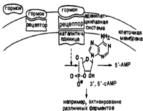
Рис.1. Механизм действия пептидных гормонов
